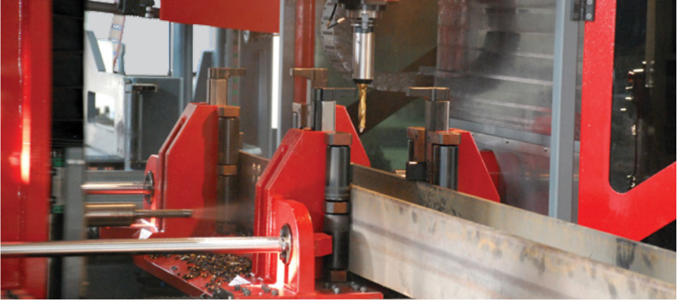
Through 3 independent spindle units on 3 ADM model, the profile can be drilled from 3 sides at the same time. Aynı bağımsız spindle ünitesi sayesinde profilin üç tarafına aynı anda delik delinebilir
